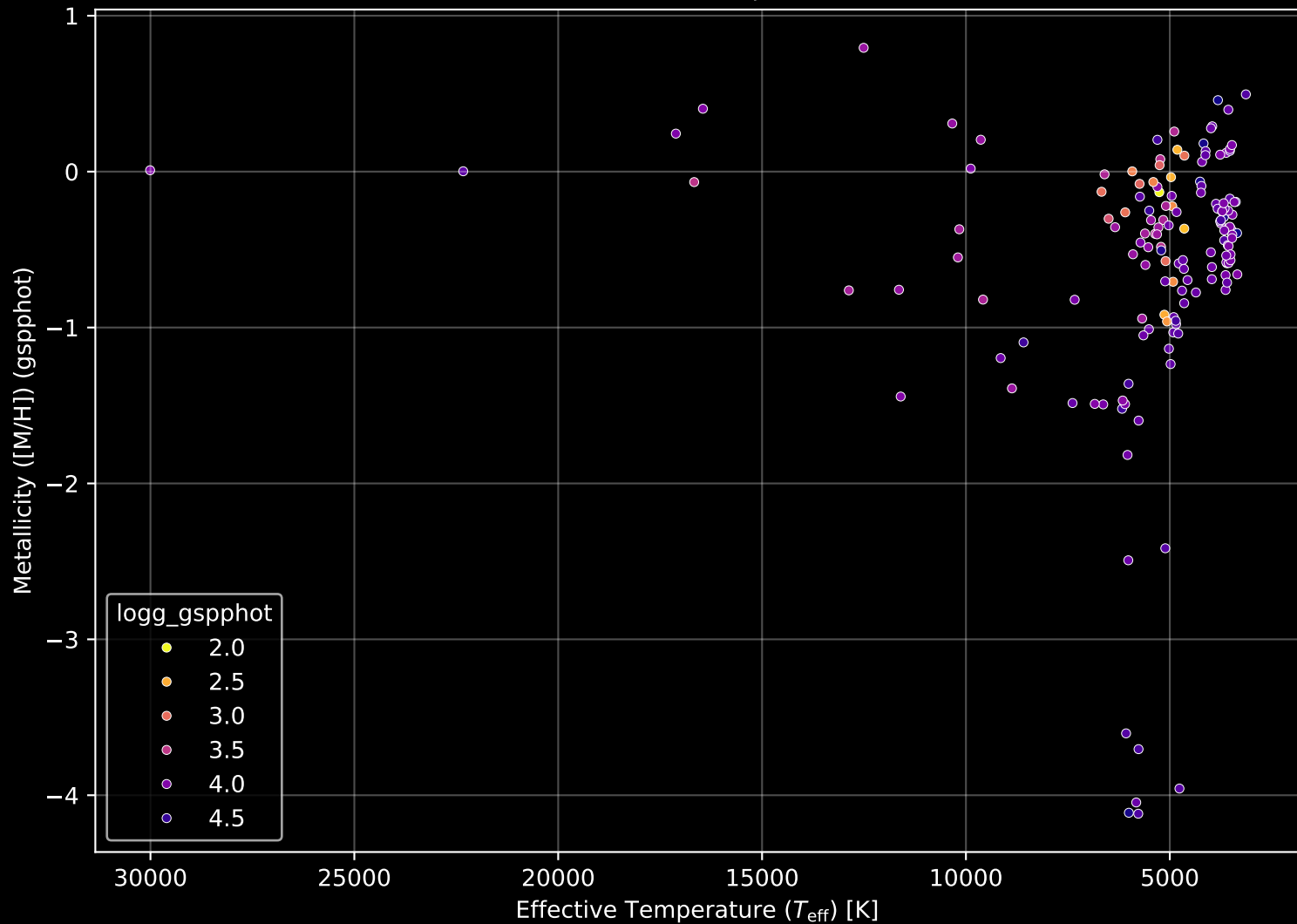
APOGEE DR17 Field: [N2264] Stellar Population Parameters (n= 152)
